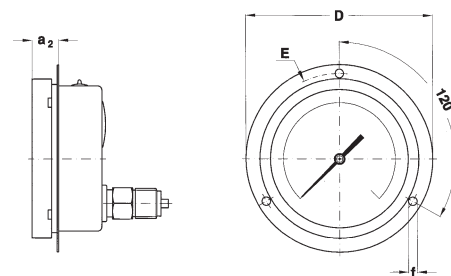
E - BRIDA ANTERIOR para racord posterior
